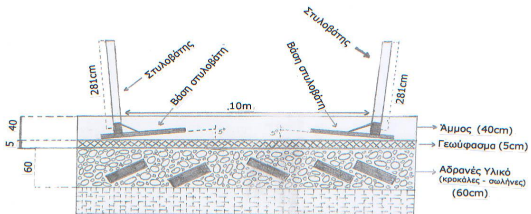
Εγκάρσια Τομή Αγωνιστικού Χώρου
